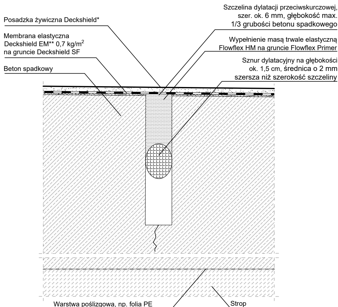
Rysunek schematyczny
