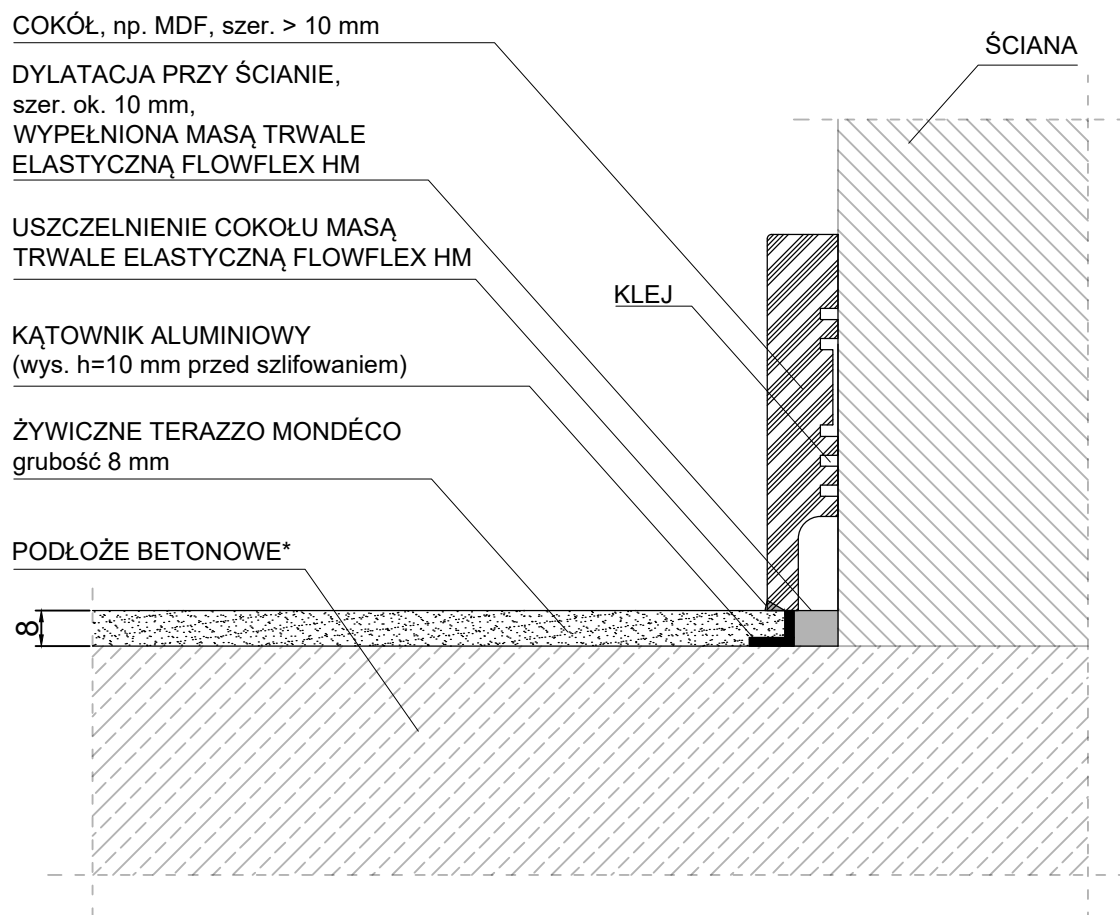
Rysunek schematyczny
