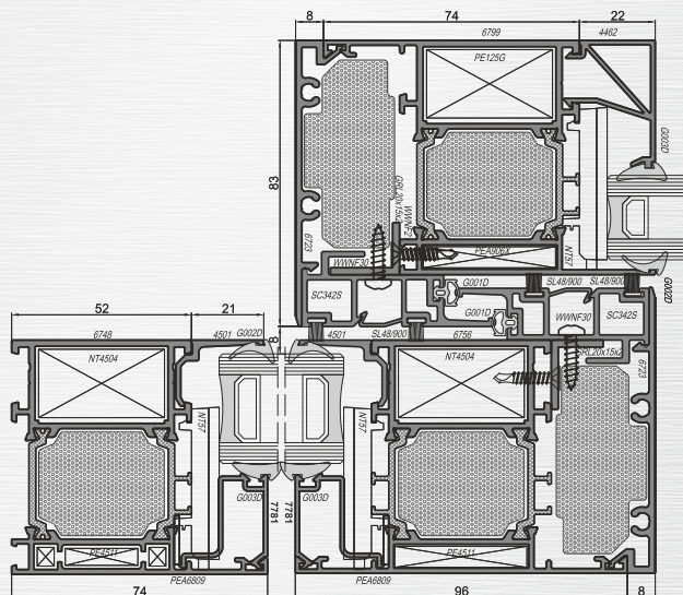
Przekrój poziomy
